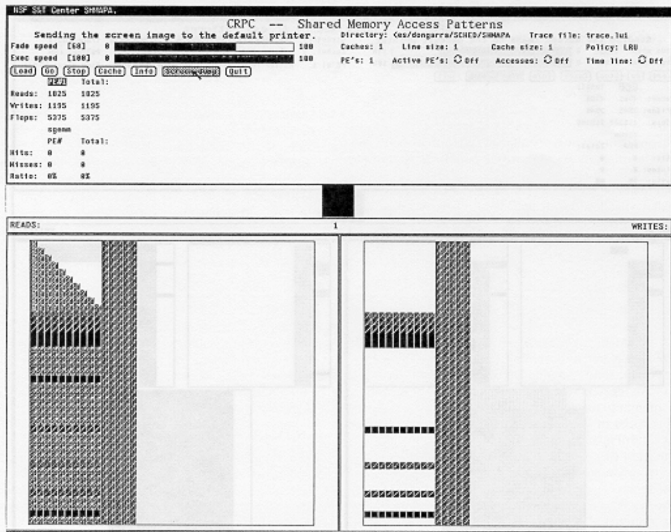
FIG. 1. LU decomposition.
